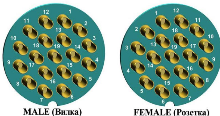
Схема расположения номеров контактов разъема Socarex и их назначение
